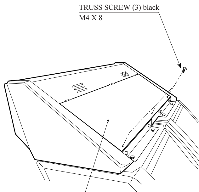
BILLBOARD LID
